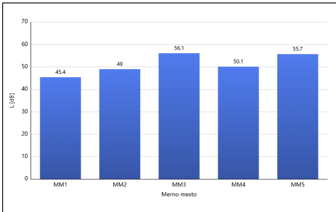
Grafik 5.8. - Večernji period merenja - Ekvivalentni nivoi buke - decembar 2024. godine
