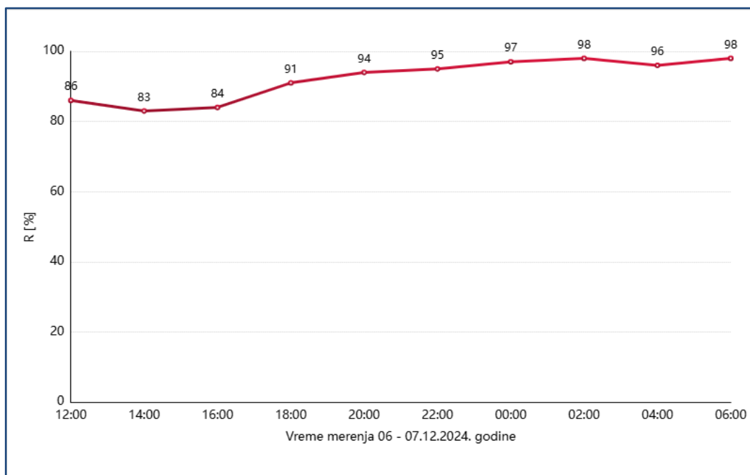
Slika 2.2. Relativna vlažnost vazduha - Ruma - decembar 2024. godine
