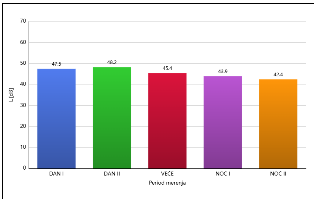
Grafik 5.1. - MM 1 ekvivalentni nivo buke za sve periode merenja - decembar 2024. godine
