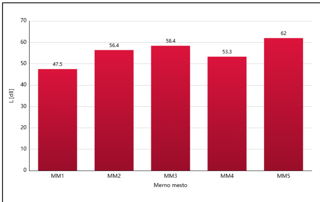
Grafik 5.6. - Dnevni period merenja 1 - Ekvivalentni nivoi buke - decembar 2024. godine
