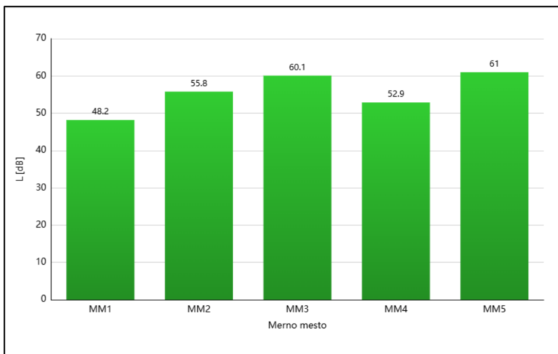
Grafik 5.7. - Dnevni period merenja 2 - Ekvivalentni nivoi buke - decembar 2024. godine
