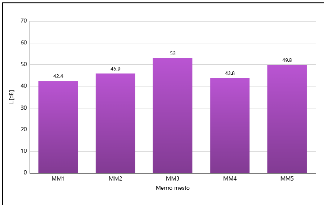
Grafik 5.10. - Noćni period merenja 2 - Ekvivalentni nivoi buke - decembar 2024. godine
