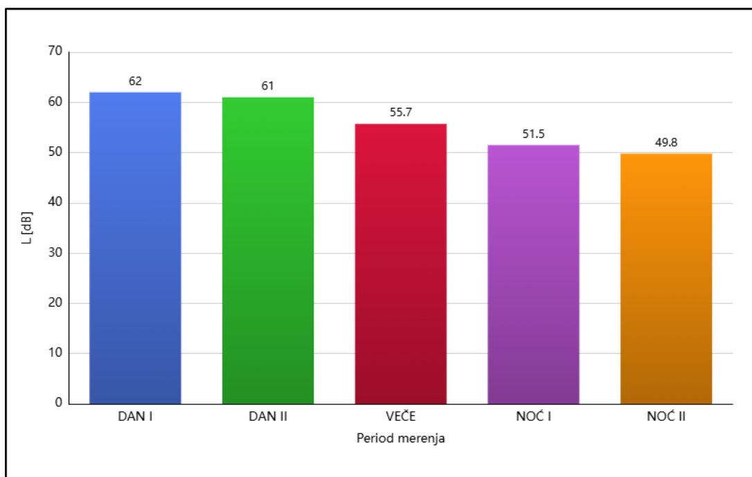
Grafik 5.5. - MM 5 ekvivalentni nivo buke za sve periode merenja - decembar 2024. godine
