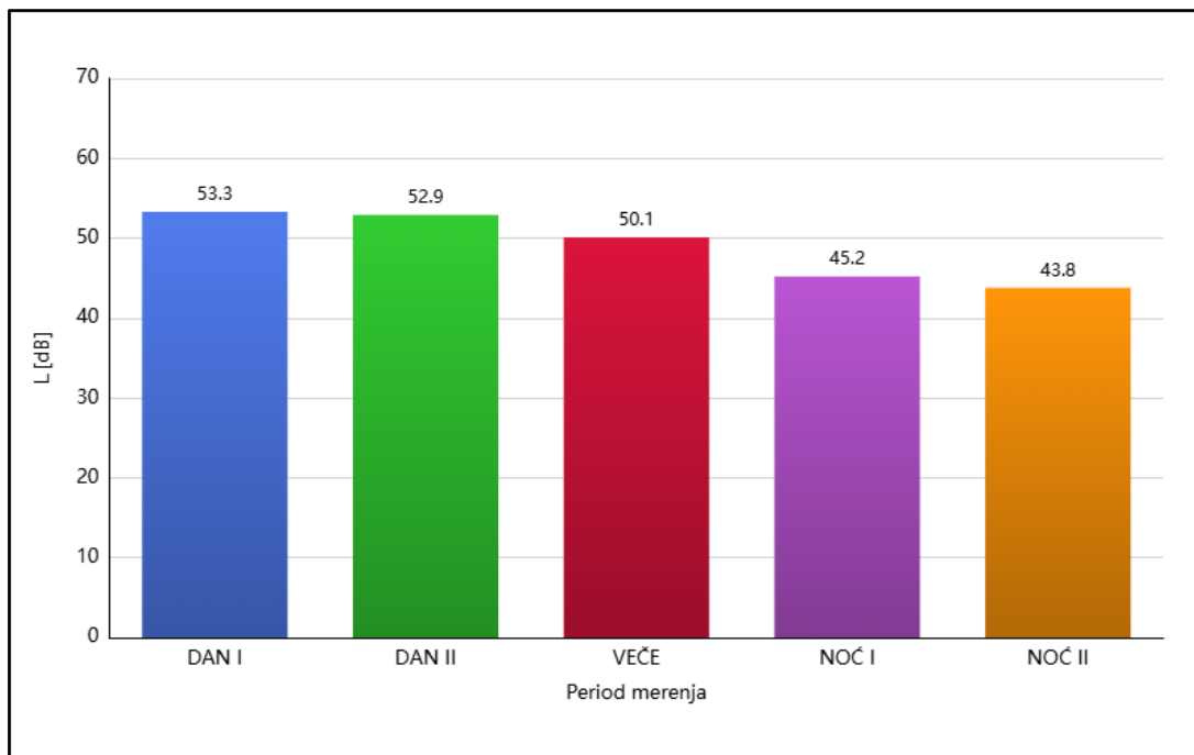
Grafik 5.4. - MM 4 ekvivalentni nivo buke za sve periode merenja - decembar 2024. godine
