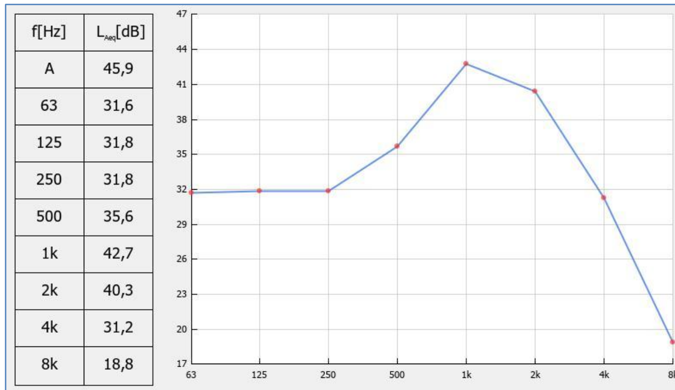
MM2 - Noćno merenje 2 - rezultati merenja
