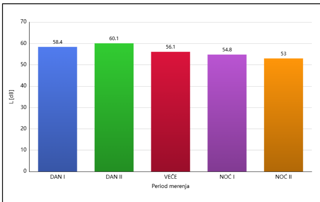
Grafik 5.3. - MM 3 ekvivalentni nivo buke za sve periode merenja - decembar 2024. godine
