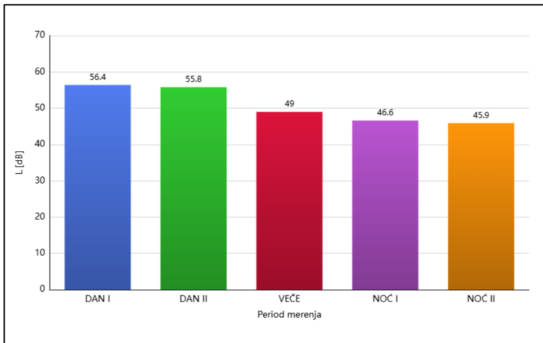
Grafik 5.2. - MM 2 ekvivalentni nivo buke za sve periode merenja - decembar 2024. godine
