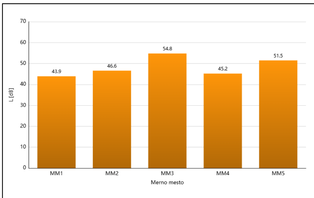
Grafik 5.9. - Noćni period merenja 1 - Ekvivalentni nivoi buke - decembar 2024. godine
