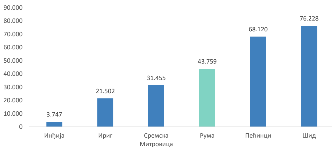
Илустрација 5: Сремска област – просечна дрвна запремина ( m^3 ), 2018. година
